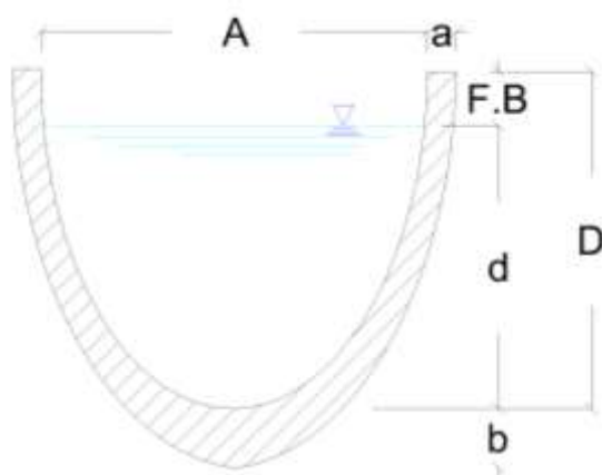
شکل (۴-۴): مقطع تیپ کانالت
