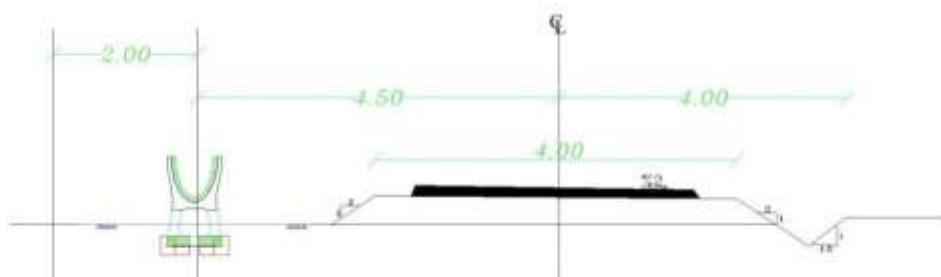
شکل (۳-۴): حریم کانالت و جاده سرویس آن
