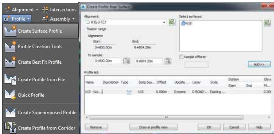
شکل (۹-۶): انتخاب سطح و مسیر برای پروفیل طولی
