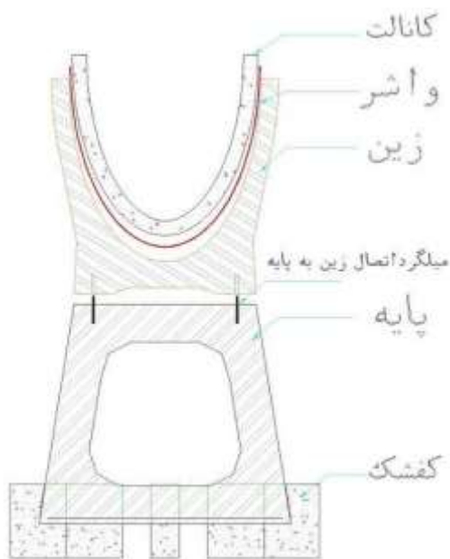
شکل (۱-۱): کانالت و متعلقات آن
