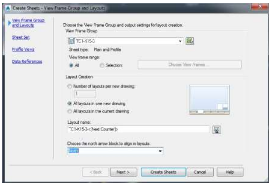
شکل (۳۱-۶): تعیین View Frame برای ساخت شیت های و محل قرارگیری شیت ها
