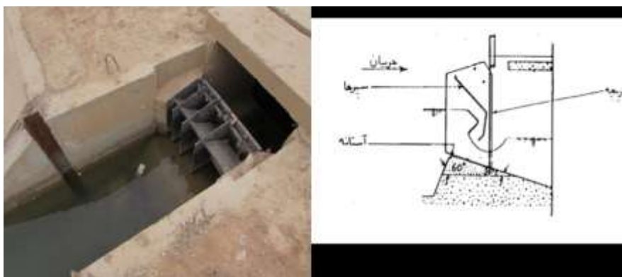
شکل (۲-۶) مشخصات و تصویر یک مدول نیرپیک دوسپره
