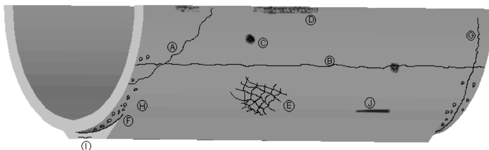
شکل (۳-۱۸): عیوب متداول در کانال‌های پیش‌ساخته بتنی
